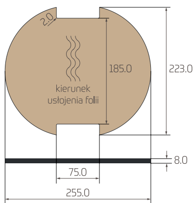
Półka dekoracyjna OVELO
