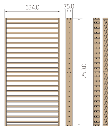
Żaluzja pozioma 75x634x1250
