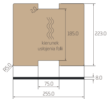
Półka dekoracyjna BOX
