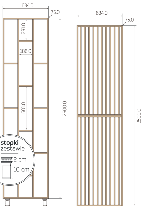
Regał dekoracyjny 75x634x2500
