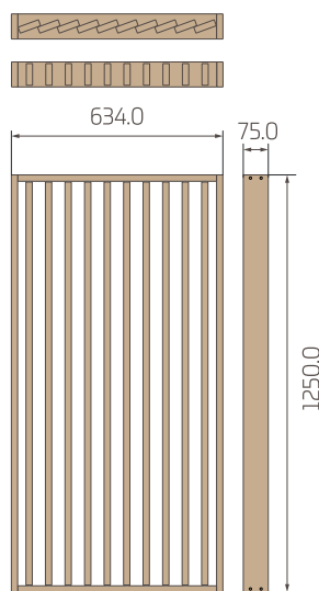
Żaluzja pionowa 75x634x1250
